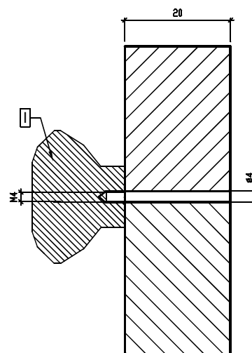
Przekrój A-A
