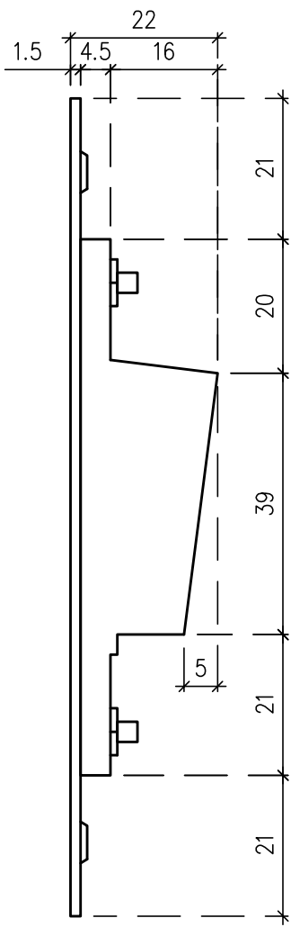
Widok z boku element II
