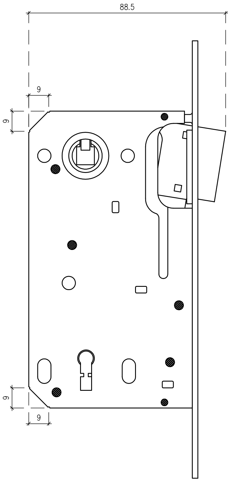
Widok z lewej strony element I
