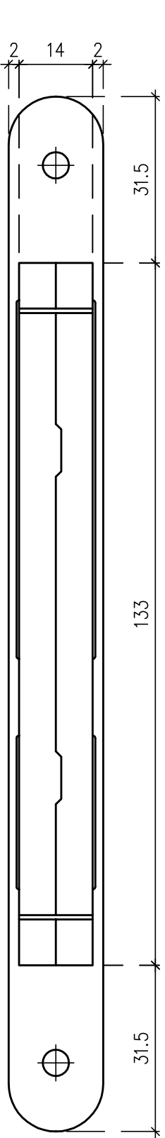
Widok z tyłu element I
