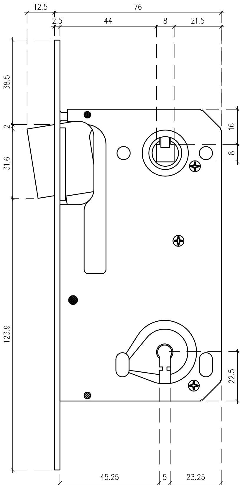
Widok z przodu element II
