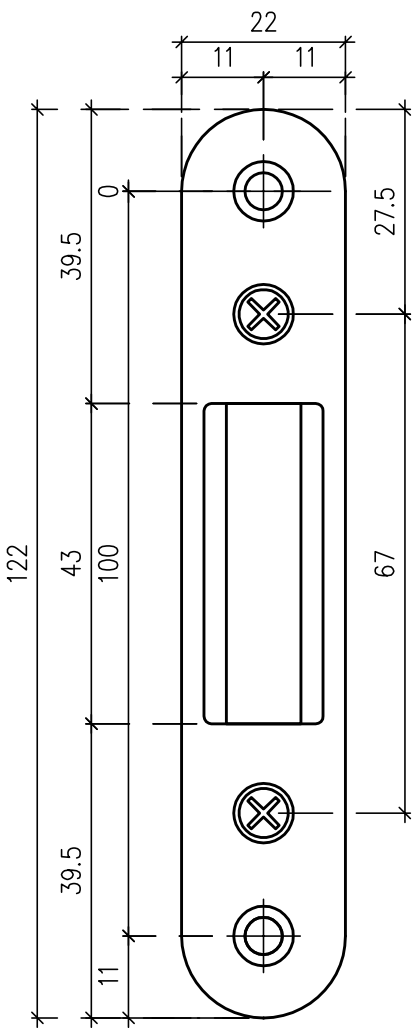
Widok z przodu element II
