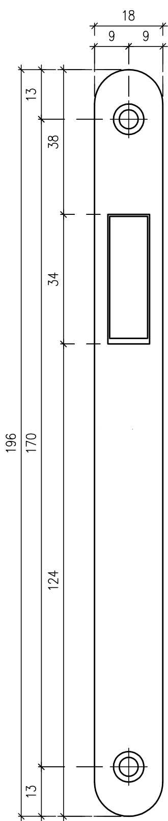
Widok z przodu element I
