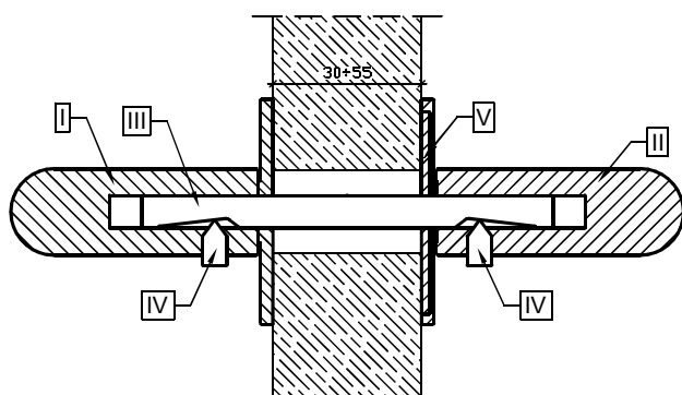
Schemat montażu elementów Przekrój A-A
