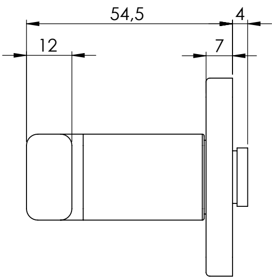
Widok z prawej Klamka I
