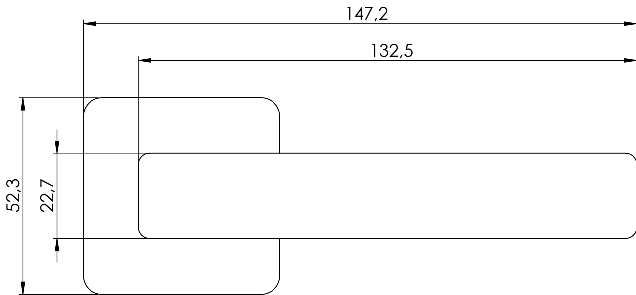
Widok z przodu Klamka I
