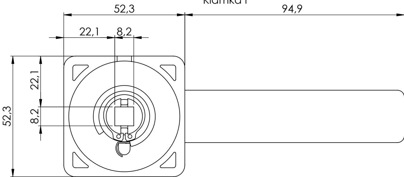
Widok z tyłu Klamka I
