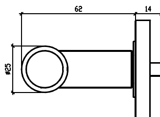
Widok z prawej strony klamka I
