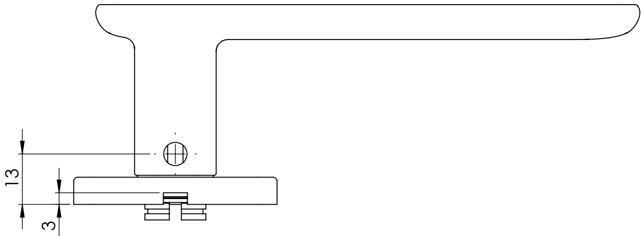
Widok z dołu Klamka I
