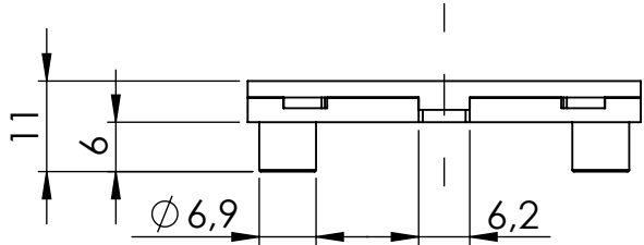
Widok z dołu Rozeta montażowa II
