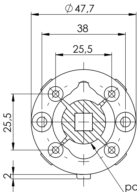
Widok z przodu Rozeta montażowa II
