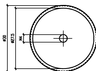
Widok z tyłu uchwyt I
