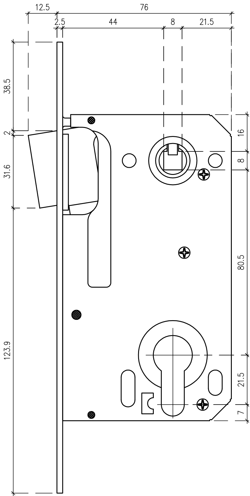
Widok z przodu element II
