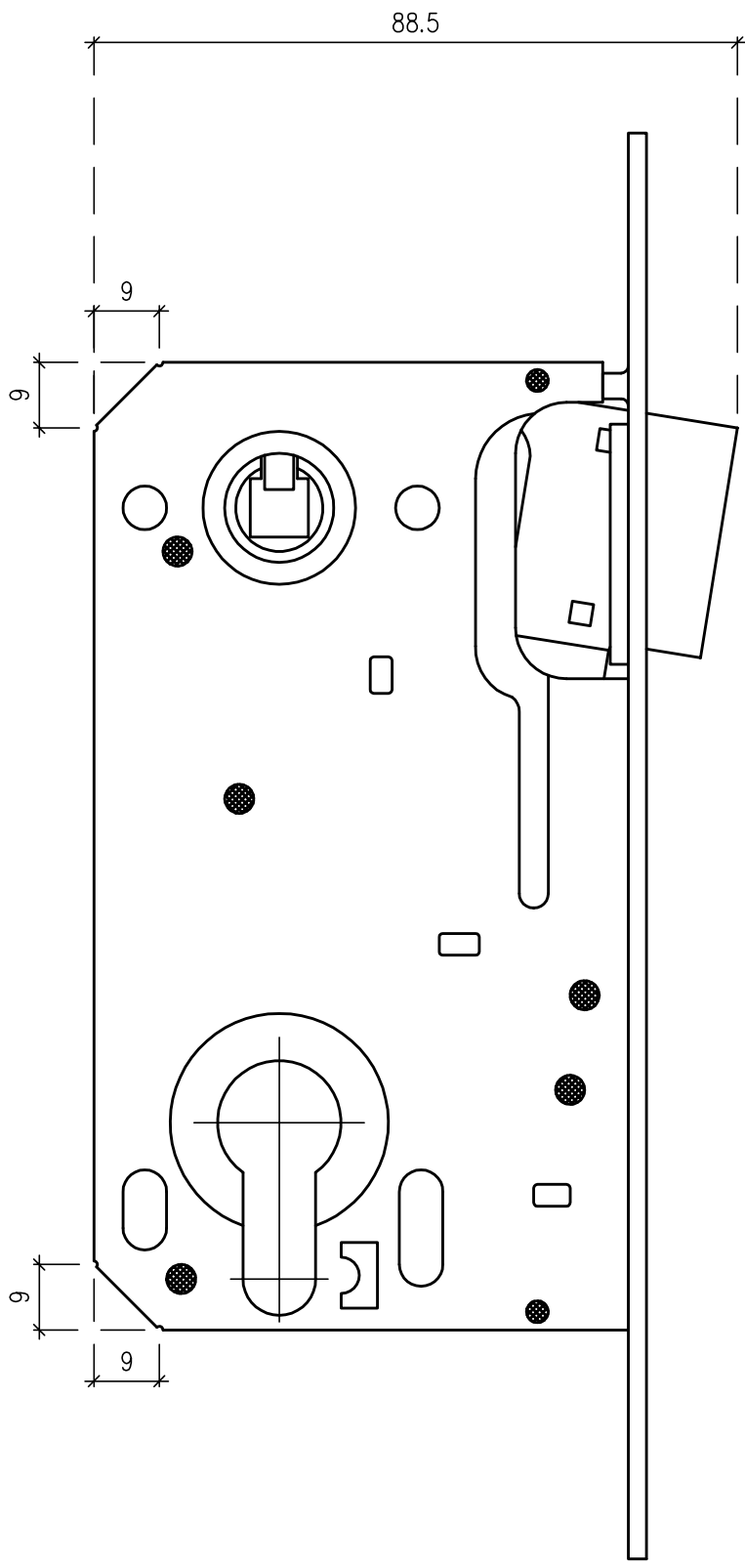
Widok z boku element II
